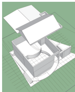
環形緩坡概念設計；其屋頂打開上視內部空間
